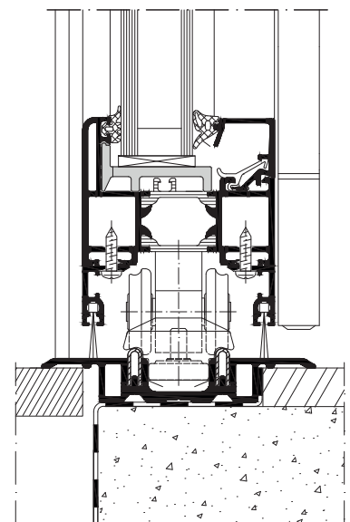
Schüco ASS 70 FD, scale 1:2 Schüco ASS 70 FD, Maßstab 1:2
