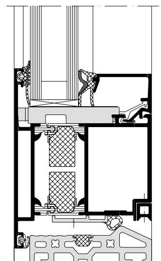
Schüco door system ADS 75 HD.HI, Sill, scale 1:2 Schüco Türsystem ADS 75 HD.HI, Fußpunkt, Maßstab 1:2
